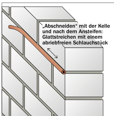
Bild 16: Fugenglattstrich
